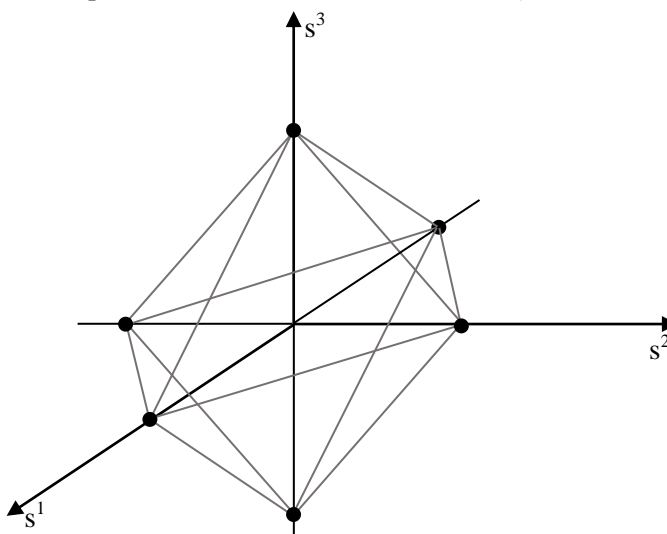
Рис. 5. Разбиение двойственного пространства на области, отвечающие дискретным значениям.
